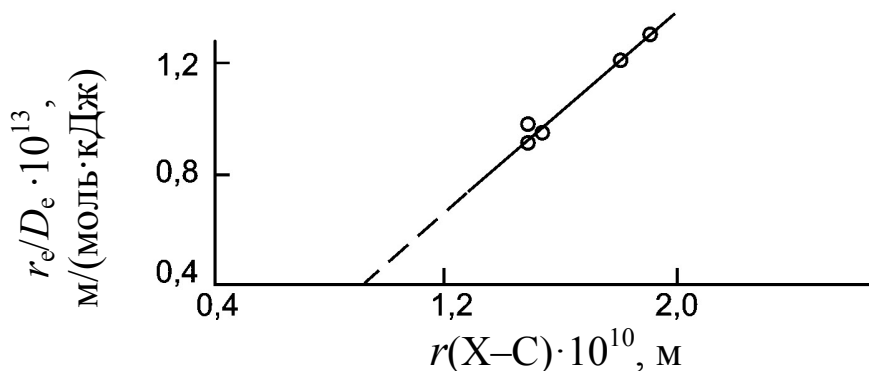
Рис. 8.3. Сравнение величин r_e/D_e r_e и r(X-C) для реакций присоединения радикалов к олефинам
