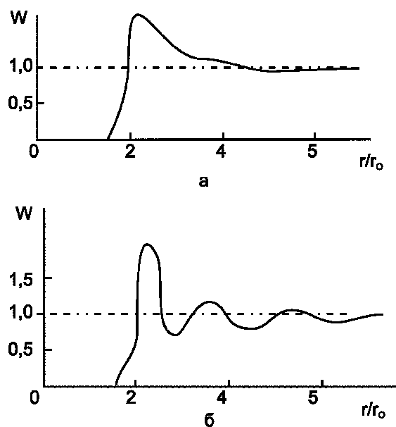
Рис. 3.1. Функция плотности W распределения частиц в зависимости от расстояния r/r_0 : а — в газе; б — в жидкости ( r_0 — радиус частицы)
