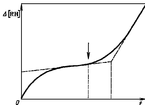
Рис. 17.2. Кинетическая кривая цепной реакции при выключении ( t = 0 ) и включении света (момент отмечен стрелкой) в методе фотохимического последействия (при больших t ), что позволяет найти k_t' , экстраполируя асимптотическую прямую накопления \Delta[\text{R}'\text{H}] к t = 0
